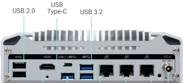
USB 2.0 USB Type-C USB 3.2 HDMI USB 3.2 2.5G LAN DC-in
