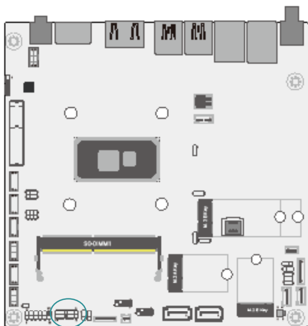
eSPI Header(Debug) (J5)
