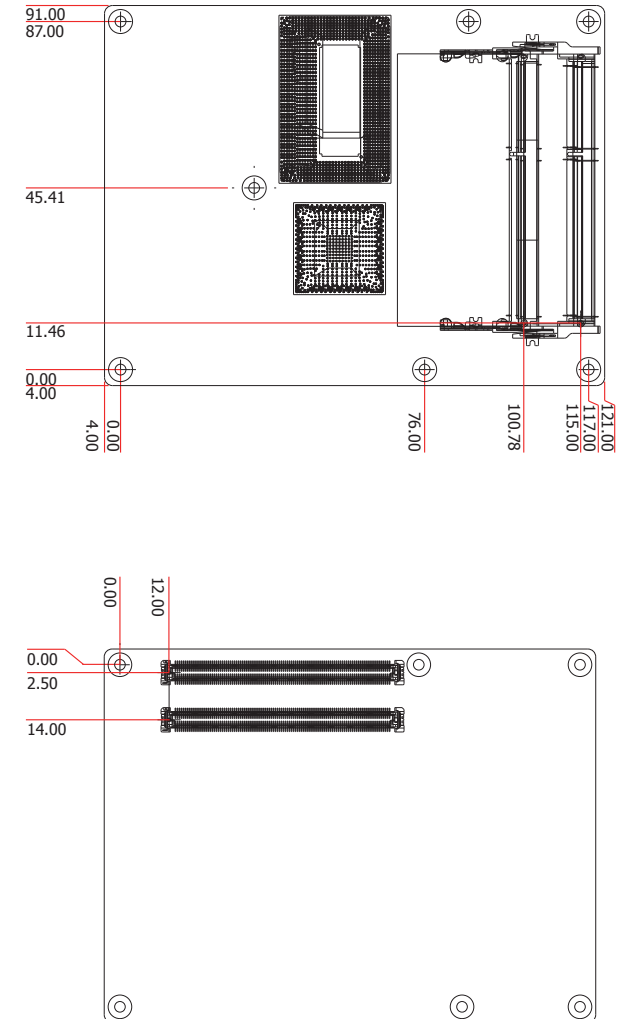
SH960-QM170/HM170 Module
